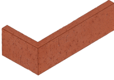
KÖŞE KAPLAMA TUĞLASI EBAT: 215 X 102 X 65 MM AĞIRLIK: 0,66 KG KULLANIM ALANI: KÖŞE DÖNÜŞLERİ, KOLON KAPLAMALARI
