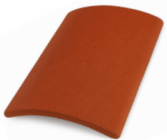
RESTORASYON KİREMİTİ EBAT: 410 X 300 X 30 MM AĞIRLIK: 7,00 KG KULLANIM ALANI: RESTORASYON ÇATI SİSTEMLERİ
